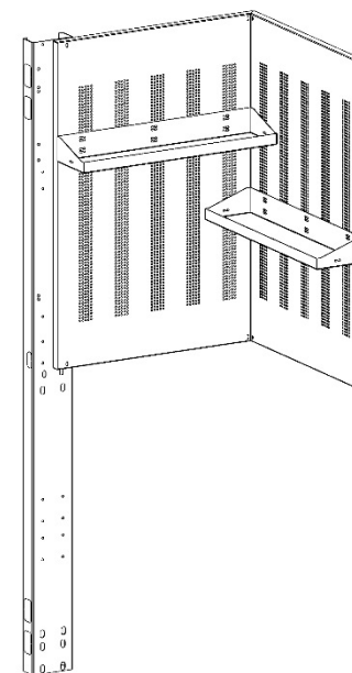
C55KAI Elemento angolare con gambe / Corner worktop 055000365
