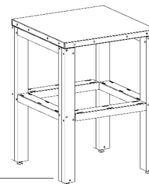
C55KAI Elemento angolare con gambe / Corner worktop 055000365
